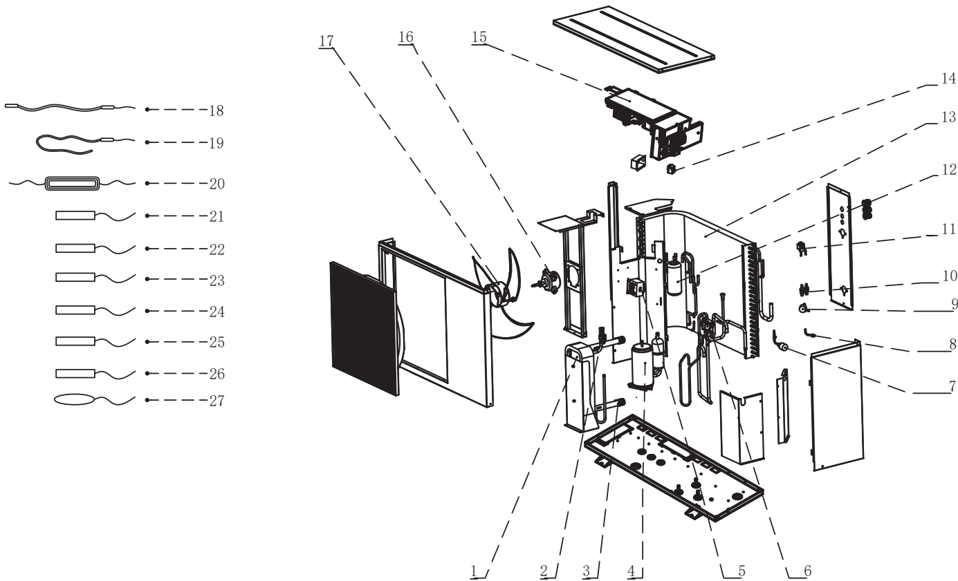
Jednostka zewnętrzna
