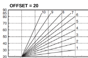
rys. 7 - Przykład przesunięcia równoległego krzywych kompensacji
