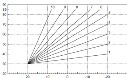
rys. 6 - Krzywe kompensacji
