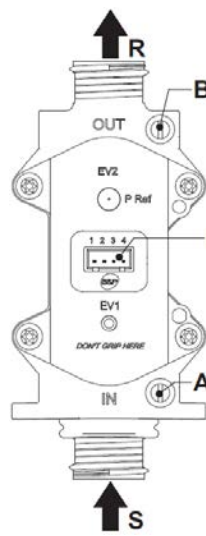
rys. 11 - Zawór gazowy
