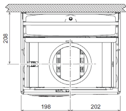
rys. 19 - Widok z góry - DIVATech D LN C30
