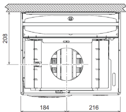
rys. 17 - Widok z góry - DIVATech D LN C24
