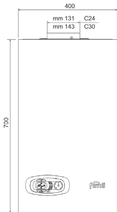
rys. 15 - Widok z przodu
