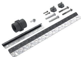
Zestaw do montażu naściennego ref. 646 099
